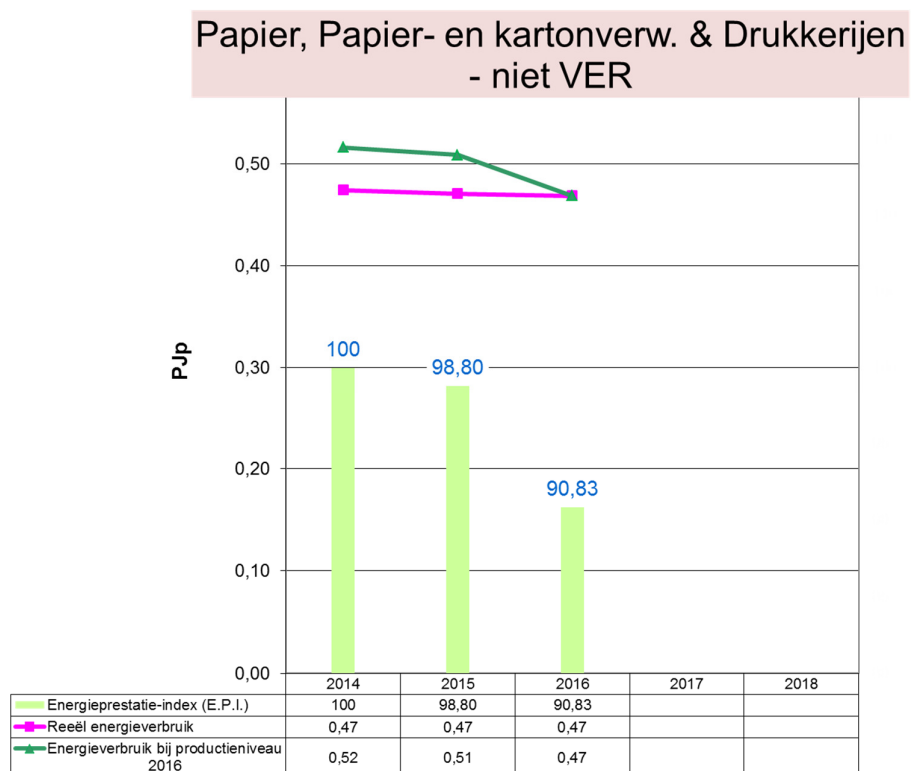
Grafiek 35: Evolutie 2014 – 2016 van het energieverbruik en de E.P.I. voor Papier, Papier- en kartonverwerking & Drukkerijen (niet VER-bedrijven)
