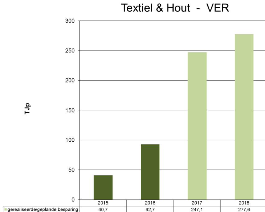
Grafiek 18: Gerealiseerde (donkergekleurd)/geplande (lichtgekleurd) besparingen Textiel & Hout (VER en niet VER-bedrijven)
