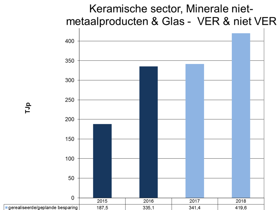
Grafiek 20: Gerealiseerde (donkergekleurd)/geplande (lichtgekleurd) besparingen Keramische sector, Minerale niet-metaalproducten & Glas (VER en niet VER-bedrijven)
