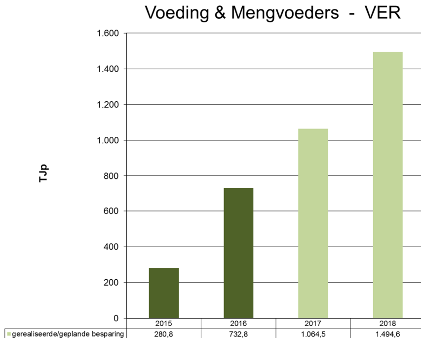
Grafiek 12: Gerealiseerde (donkergekleurd)/geplande (lichtgekleurd) besparingen Voeding & Mengvoeders (VER-bedrijven)
