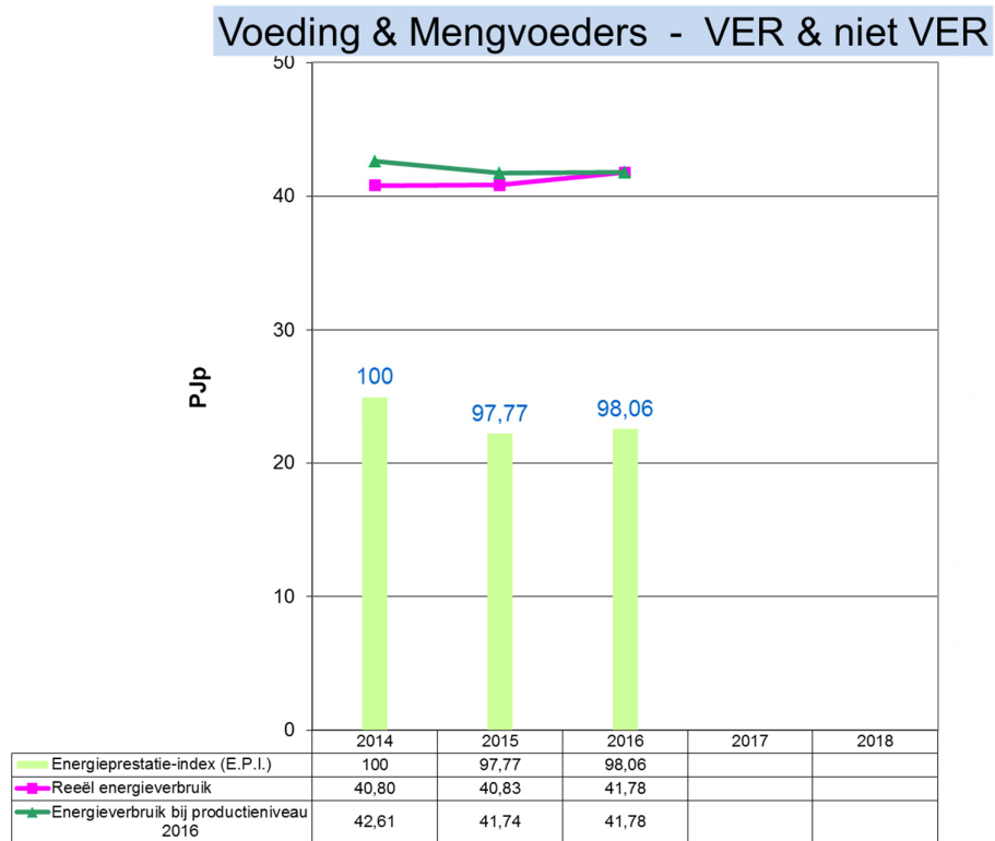
Grafiek 36: Evolutie 2014 – 2016 van het energieverbruik en de E.P.I. voor Voeding & Mengvoeders (VER en niet VER-bedrijven)
