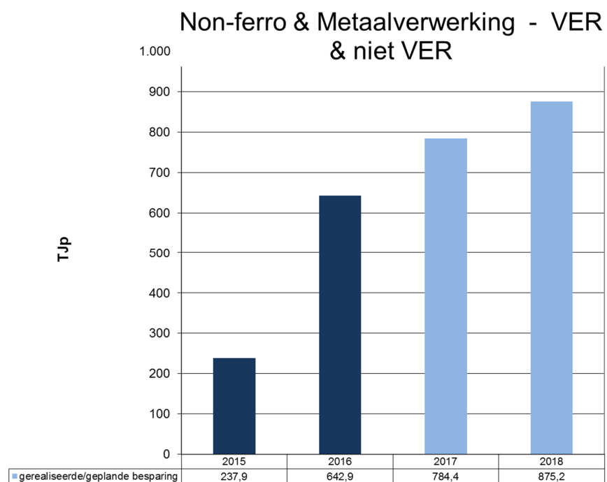
Grafiek 14: Gerealiseerde (donkergekleurd)/geplande (lichtgekleurd) besparingen Non-ferro & Metaalverwerking (VER en niet VER-bedrijven)
