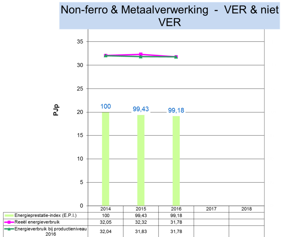
Grafiek 39: Evolutie 2014 – 2016 van het energieverbruik en de E.P.I. voor Non-ferro & Metaalverwerking (VER en niet VER-bedrijven)
