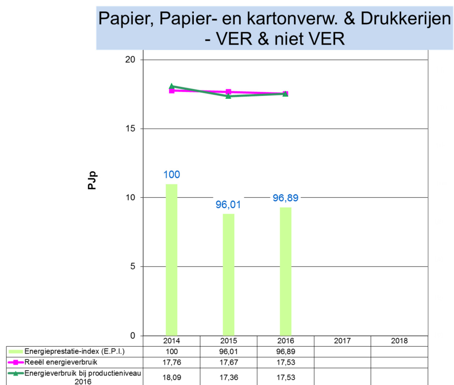
Grafiek 33: Evolutie 2014 – 2016 van het energieverbruik en de E.P.I. voor Papier, Papier- en kartonverwerking & Drukkerijen (VER en niet VER-bedrijven)
