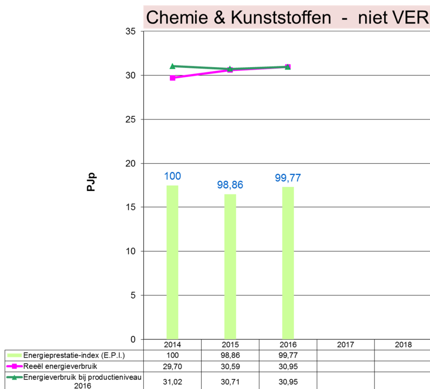
Grafiek 31: Evolutie 2014 – 2016 van het energieverbruik en de E.P.I. voor Chemie & Kunststoffen (niet VER-bedrijven)
