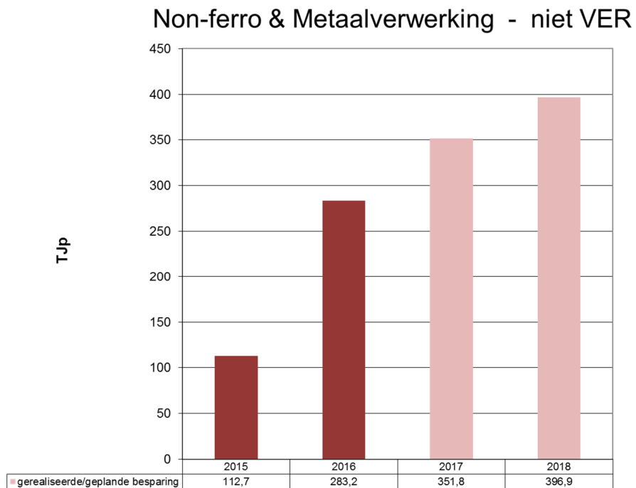
Grafiek 16: Gerealiseerde (donkergekleurd)/geplande (lichtgekleurd) besparingen Non-ferro & Metaalverwerking (niet VER-bedrijven)
