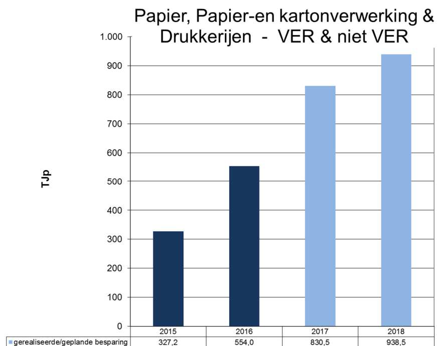
Grafiek 8: Gerealiseerde (donkergekleurd)/geplande (lichtgekleurd) besparingen Papier, Papier- en kartonverwerking & Drukkerijen (VER en niet VER-bedrijven)
