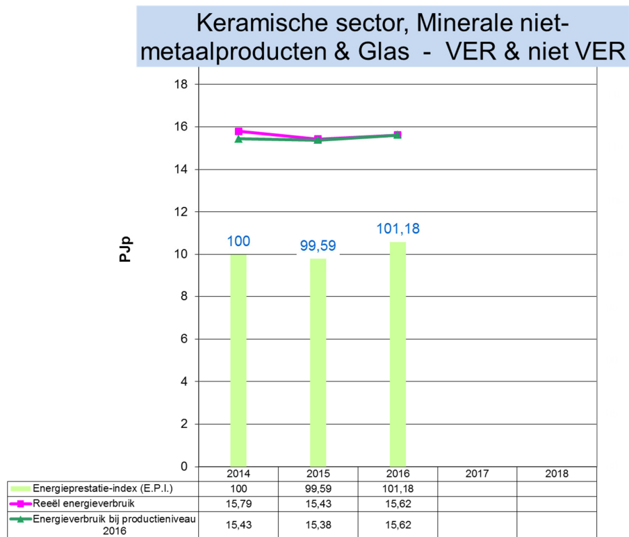
Grafiek 45: Evolutie 2014 – 2016 van het energieverbruik en de E.P.I. voor Keramische sector, Minerale niet-metaalproducten & Glas (VER en niet VER-bedrijven)
