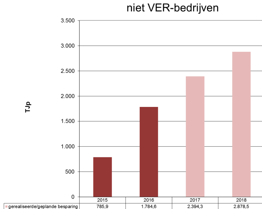
Grafiek 3: Gerealiseerde (donkergekleurd)/geplande (lichtgekleurd) besparingen (niet VER-bedrijven)
