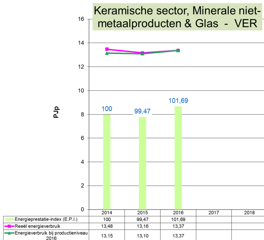
Grafiek 46: Evolutie 2014 – 2016 van het energieverbruik en de E.P.I. voor Keramische sector, Minerale niet-metaalproducten & Glas (VER-bedrijven)
