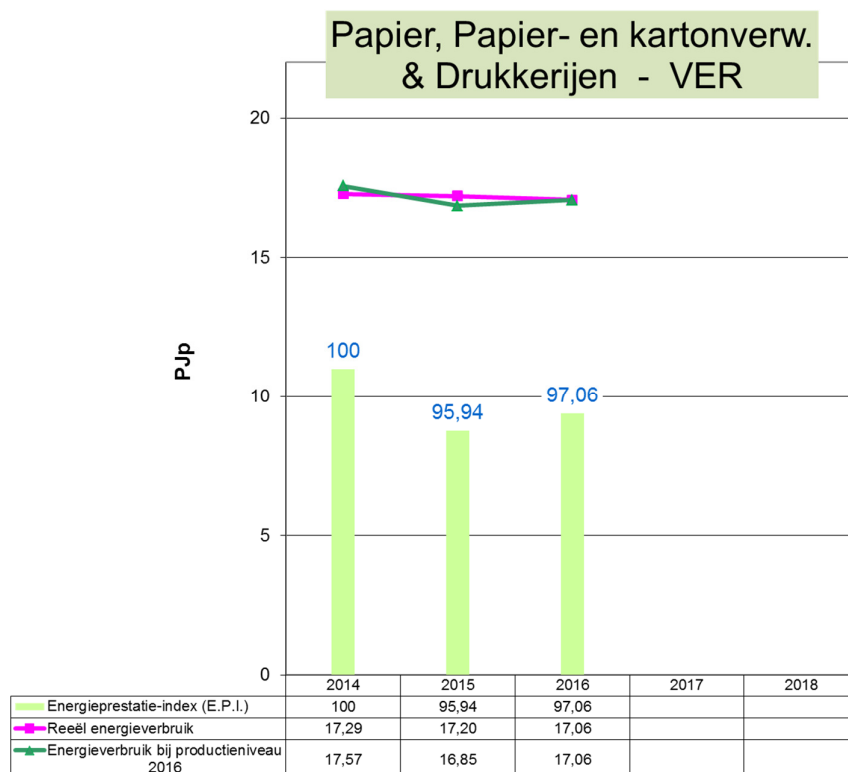
Grafiek 34: Evolutie 2014 – 2016 van het energieverbruik en de E.P.I. voor Papier, Papier- en kartonverwerking & Drukkerijen (VER-bedrijven)
