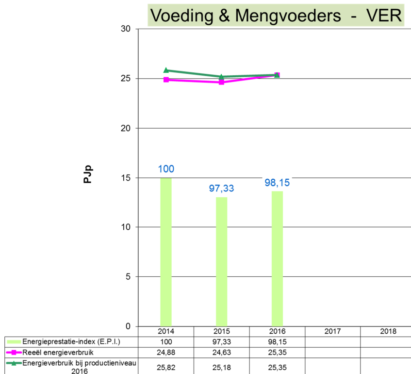
Grafiek 37: Evolutie 2014 – 2016 van het energieverbruik en de E.P.I. voor Voeding & Mengvoeders (VER-bedrijven)
