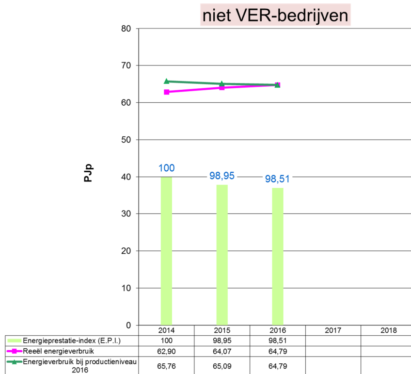
Grafiek 28: Evolutie 2014 – 2016 van het energieverbruik en de E.P.I. voor de niet VER-bedrijven
