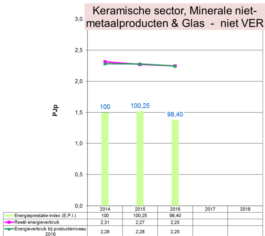
Grafiek 47: Evolutie 2014 – 2016 van het energieverbruik en de E.P.I. voor Keramische sector, Minerale niet-metaalproducten & Glas (niet VER-bedrijven)
