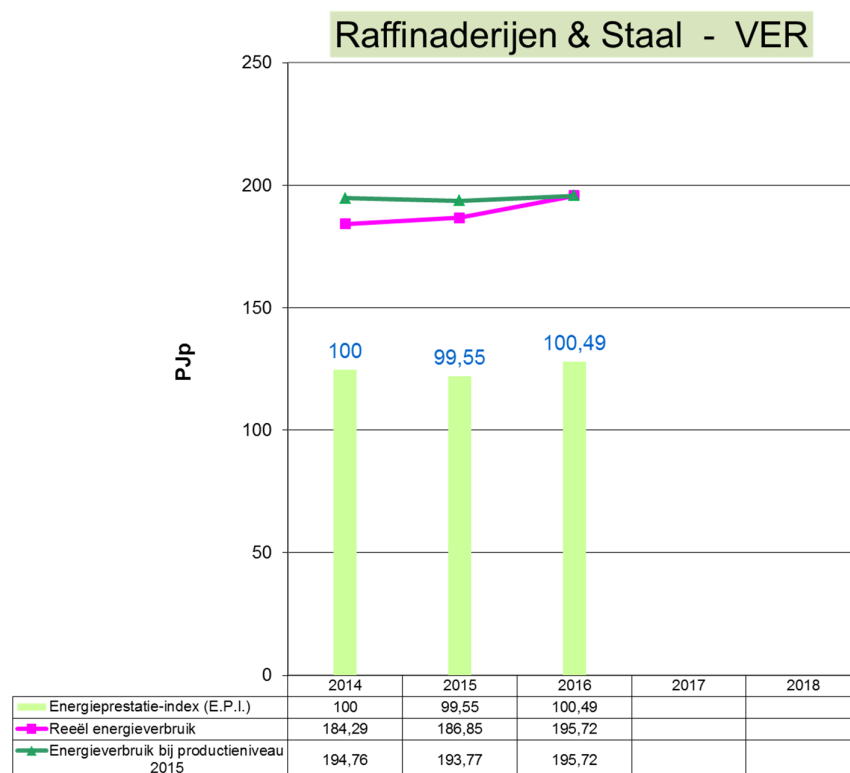
Grafiek 32: Evolutie 2014 – 2016 van het energieverbruik en de E.P.I. voor Raffinaderijen & Staal (VER-bedrijven)
