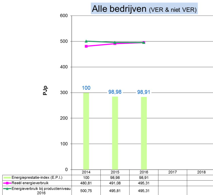
Grafiek 26: Evolutie 2014 – 2016 van het energieverbruik en de E.P.I. voor alle bedrijven
