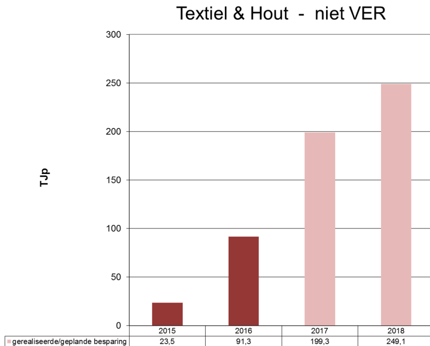
Grafiek 19: Gerealiseerde (donkergekleurd)/geplande (lichtgekleurd) besparingen Textiel & Hout (VER en niet VER-bedrijven)
