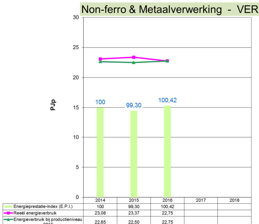
Grafiek 40: Evolutie 2014 – 2016 van het energieverbruik en de E.P.I. voor Non-ferro & Metaalverwerking (VER-bedrijven)
