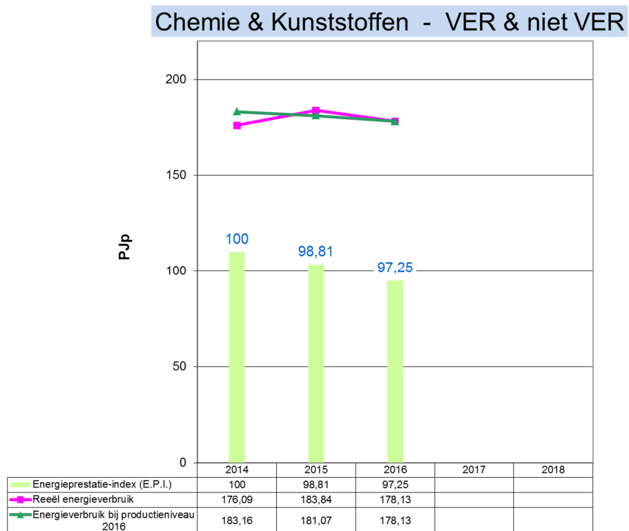
Grafiek 29: Evolutie 2014 – 2016 van het energieverbruik en de E.P.I. voor Chemie & Kunststoffen (VER en niet VER-bedrijven)
