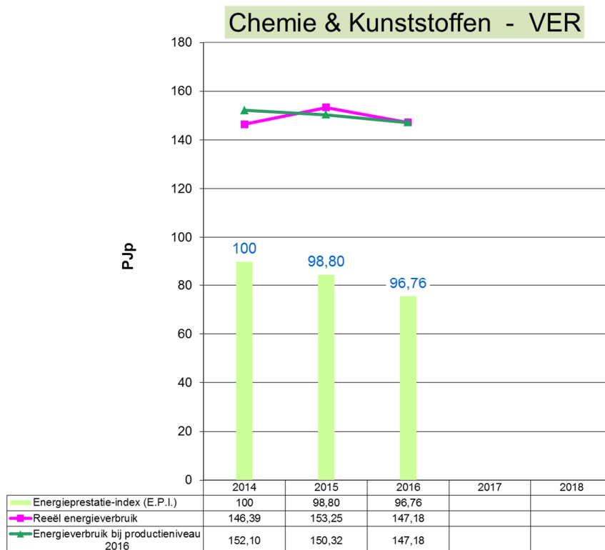
Grafiek 30: Evolutie 2014 – 2016 van het energieverbruik en de E.P.I. voor Chemie & Kunststoffen (VER-bedrijven)
