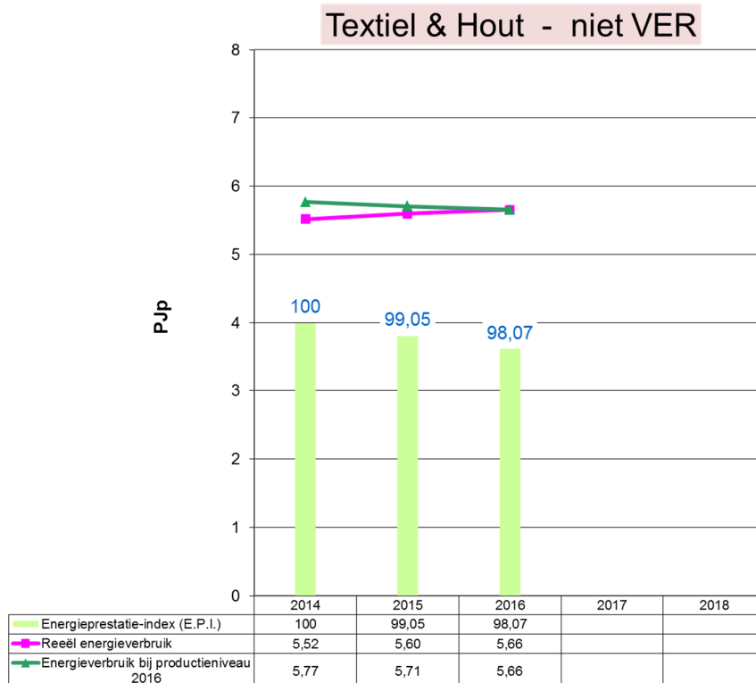
Grafiek 44: Evolutie 2014 – 2016 van het energieverbruik en de E.P.I. voor Textiel & Hout (niet VER-bedrijven)
