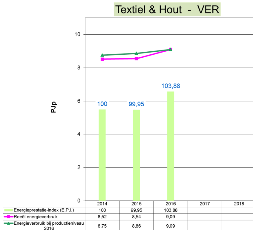
Grafiek 43: Evolutie 2014 – 2016 van het energieverbruik en de E.P.I. voor Textiel & Hout (VER-bedrijven)
