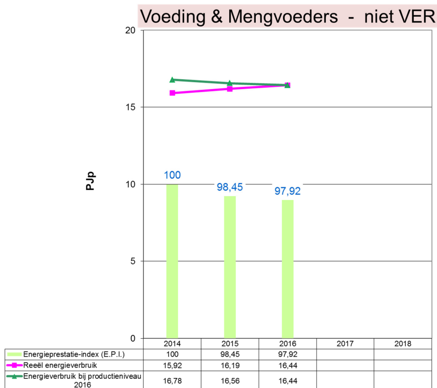
Grafiek 38: Evolutie 2014 – 2016 van het energieverbruik en de E.P.I. voor Voeding & Mengvoeders (niet VER-bedrijven)
