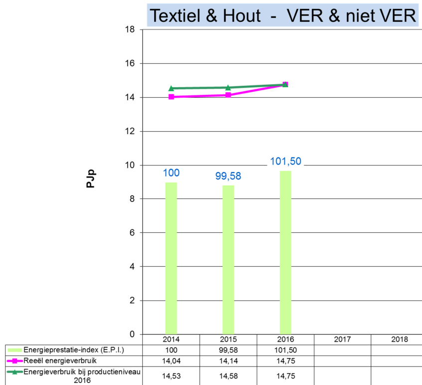
Grafiek 42: Evolutie 2014 – 2016 van het energieverbruik en de E.P.I. voor Textiel & Hout (VER en niet VER-bedrijven)
