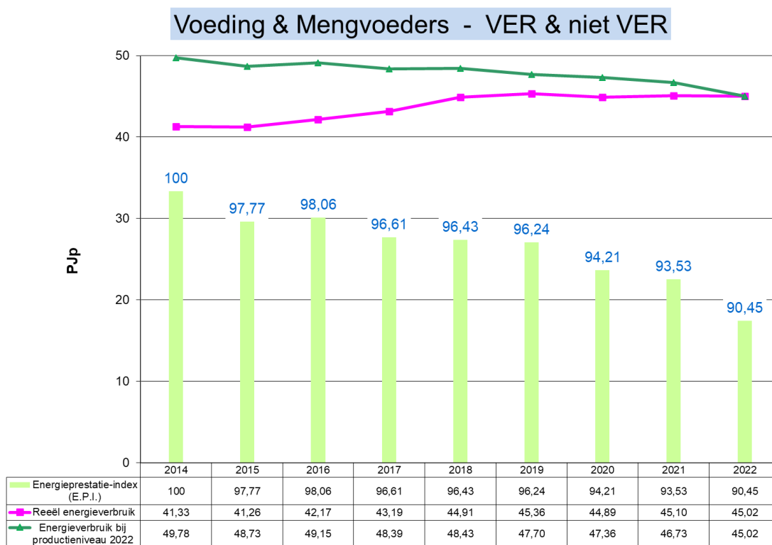
Grafiek 36: Evolutie 2014 – 2022 van het energieverbruik en de E.P.I. voor Voeding & Mengvoeders (VER en niet VER-bedrijven)
