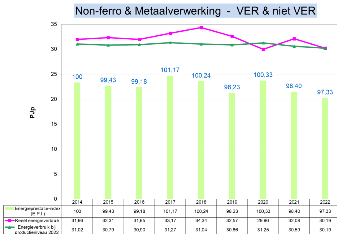
Grafiek 39: Evolutie 2014 – 2022 van het energieverbruik en de E.P.I. voor Non-ferro & Metaalverwerking (VER en niet VER-bedrijven)
